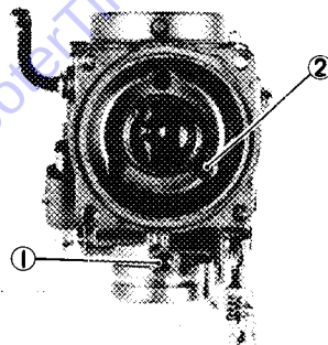
1. Vis de gicleur 2. Ralenti d'air
