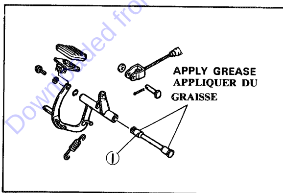
1. Arbre de pivot
