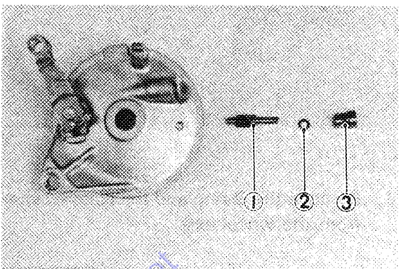
1. Meter gear 2. Washer 3. Bush 1. Pignon de compteur 2. Rondelle 3. Bague
