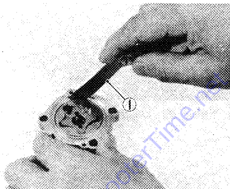
1. Jauge d'épaisseur
