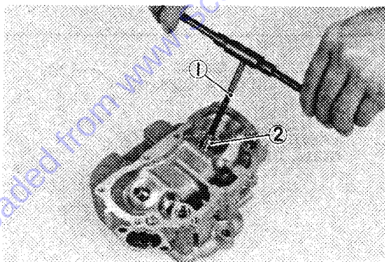
1. Alesoir 2. Guide de soupape
