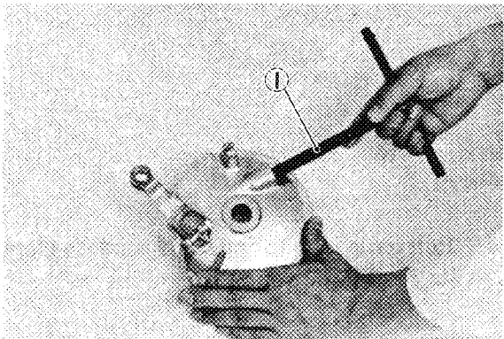
1. Meter gear bush driver (Special tool) 1. Chassoir de bague de pignon de compteur (Outil spécial)
