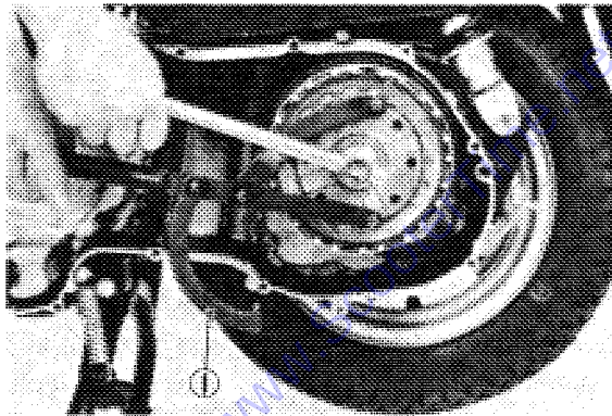
1. Poignée de rotor
