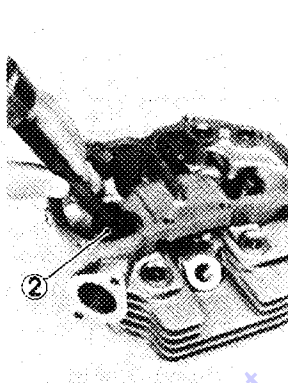
1. Outil de mise en place de guide de soupape 2. Extracteur de guide de soupape
