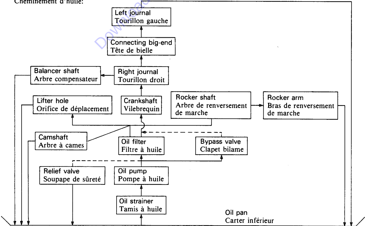
—Routes of oil: Cheminement d'huile:
