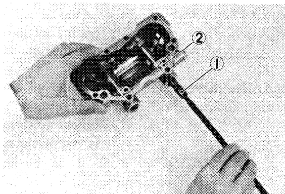
1. Trou (Axe de culbuteur) 2. Trou (Couvercle de culasse)
