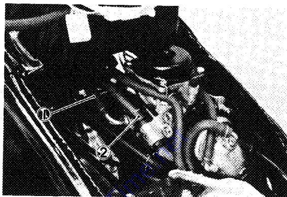
1. Tube à carburant 2. Tube de starter
