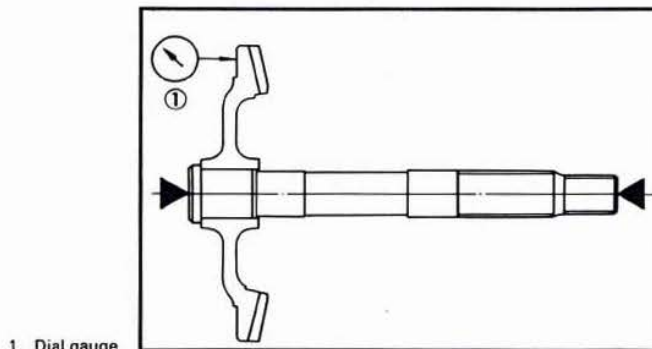
1. Comparateur à cadran
